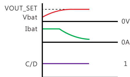
充電電壓設定大於電池電壓且C/D=1
