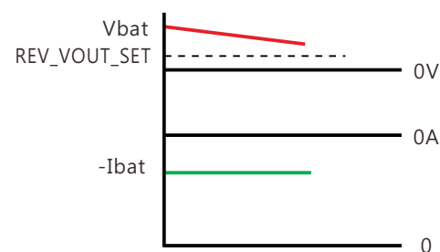
放電電壓設定小於電池電壓且C/D=0
