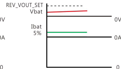
放電電壓設定大於電池電壓且C/D=0
